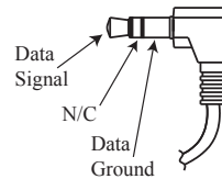
Figure 09– Data Out mini plug
